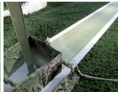
9 | Verklebung der Rasenkanten mit Vliesunterlage und Zweikomponentenkleber
