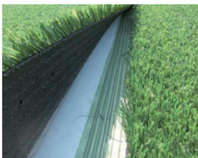
11 | Pegado del césped con el textil adhesivado de 2 componentes
