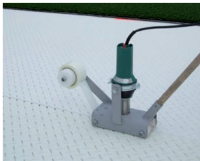
4 | Máquina móvil con cinta adhesiva para soldar los rollos
