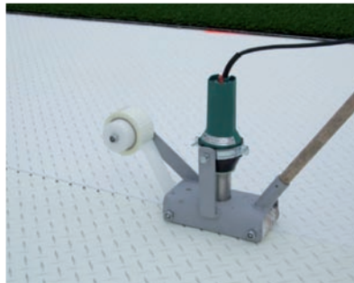
4 | Saldatrice portatile con nastro adesivo per saldare i rotoli
