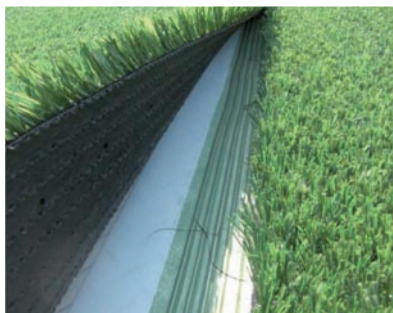
11 | Laminazione dell'erba con nastro e adesivo bicomponente
