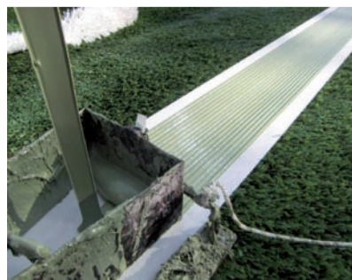
9 | Нанесение на дерн слоя ворса и 2-компонентного клея
